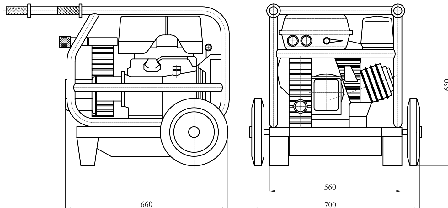
PRZYKŁADOWA FORMA ZABUDOWY ZASILACZA W WYKONANIU Z SILNIKIEM SPALINOWYM
